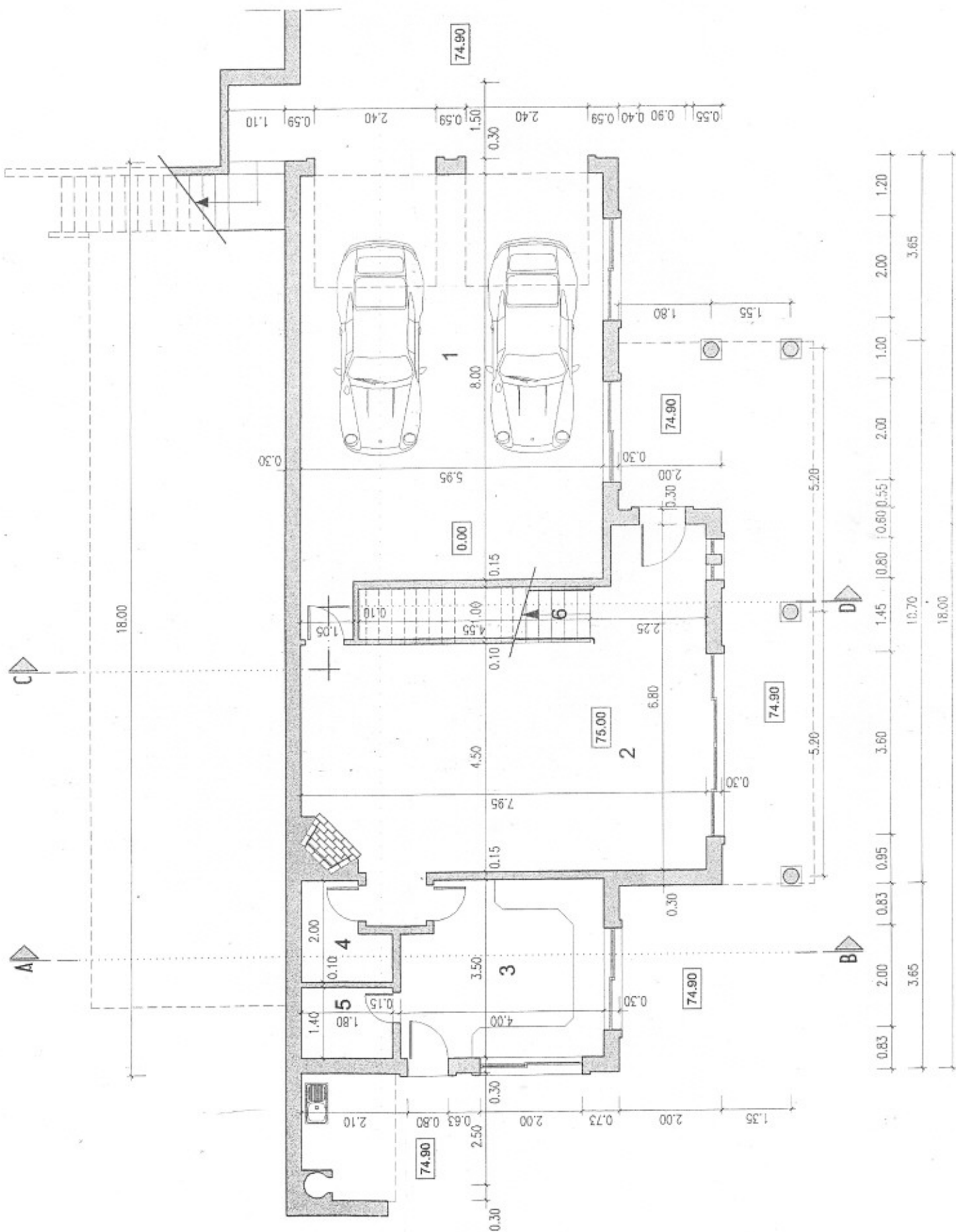
PIANTA DO RÉS DO CHÃO
