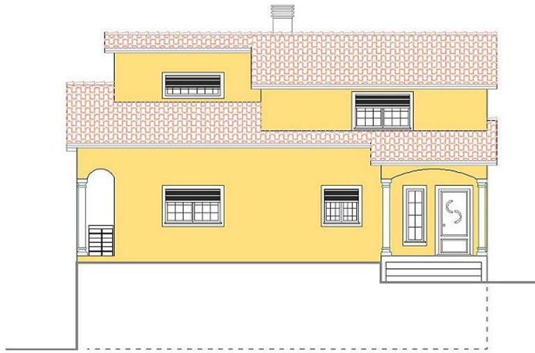
Alçado Principal
